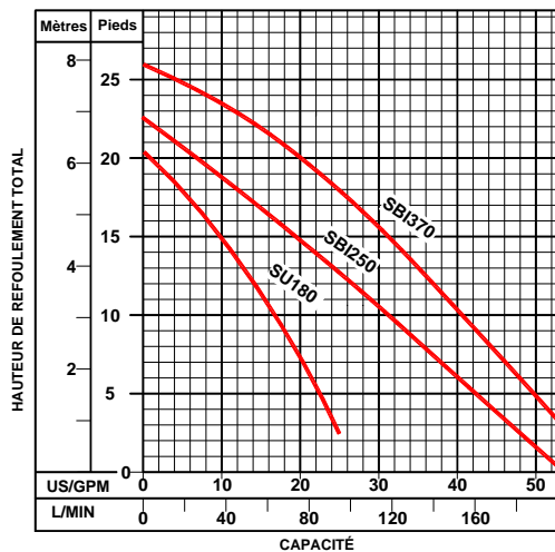
COURBE POMPAGE SÉRIE SBI / SU
