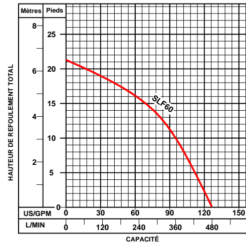
COURBE POMPAGE SÉRIE SLF
